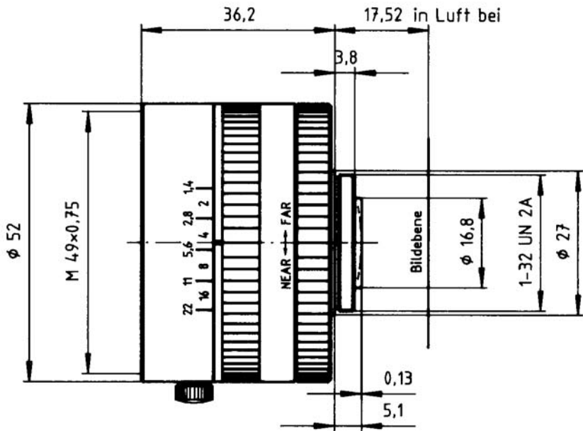
Cinegon 1,4/8 in man. Blendenkörper
